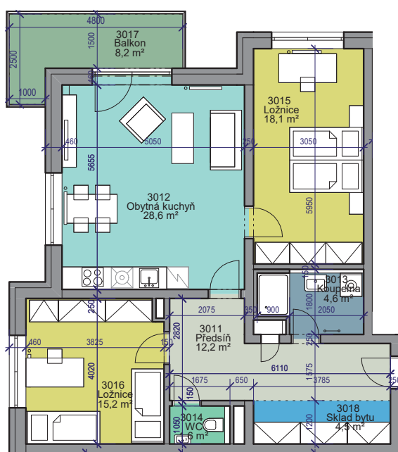
Půdorys bytu
